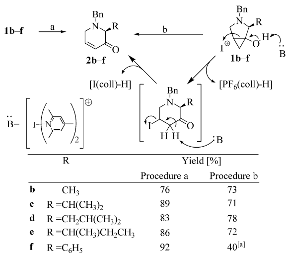
Scheme 4. (a) FeCl 3 , Et 2 O, 0 °C, 3 h, then AcONa, MeOH, 20 °C; (b) bis( sym -collidine)IPF 6 , CH 2 Cl 2 , 20 °C.
