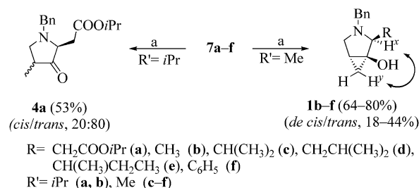
Scheme 2. (a) Ti(O i Pr) 4 (0.1 equiv.), i PrMgBr (5 equiv.), THF/Et 2 O, 20 °C.
